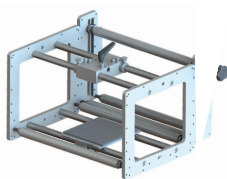
Cadre de montaj standardizate cu lățimi de până la 1.000 mm.
